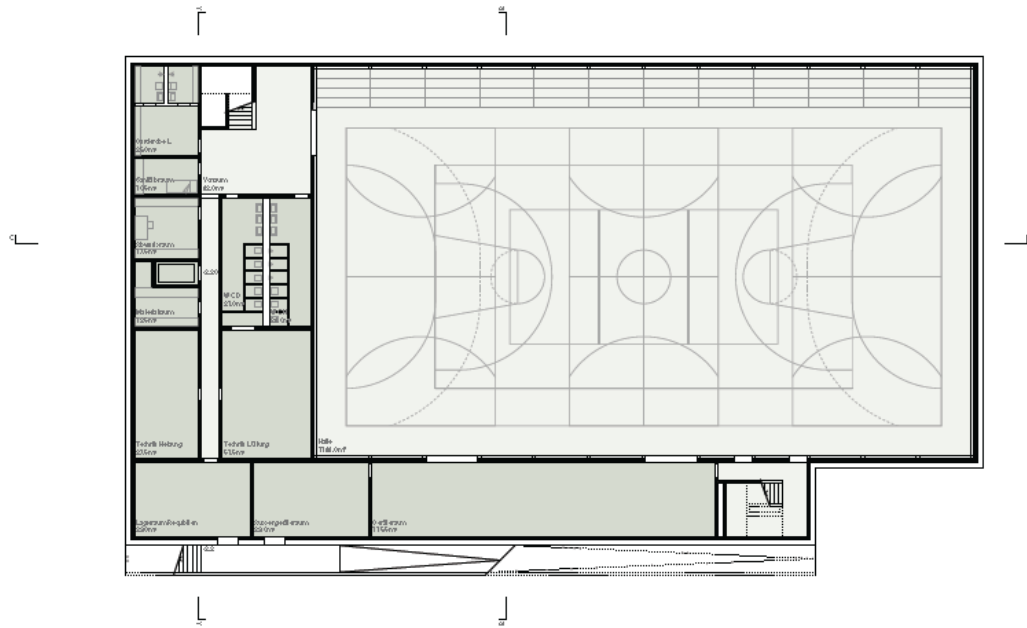
UNTERGESCHOSS M1 200
